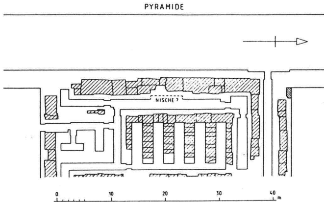
Abb.3 Der westliche Teil des Chephrentempels (nach MARAGIOGLIO/RINALDI, L'architettura V, Tf. 11 Fig.1)
