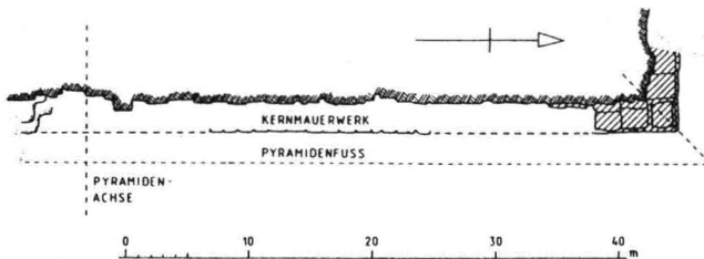
Abb.2 Die Ostseite der Djedefrepyramide (nach MARAGIOGLIO/RINALDI, L'architettura V, Tf.4 Fig.4)
