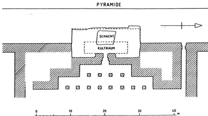
Abb.1 Der westliche Teil des Cheopstempels (nach MARAGIOGLIO/RINALDI, L'architettura IV, Tf. 9 Fig.1)
