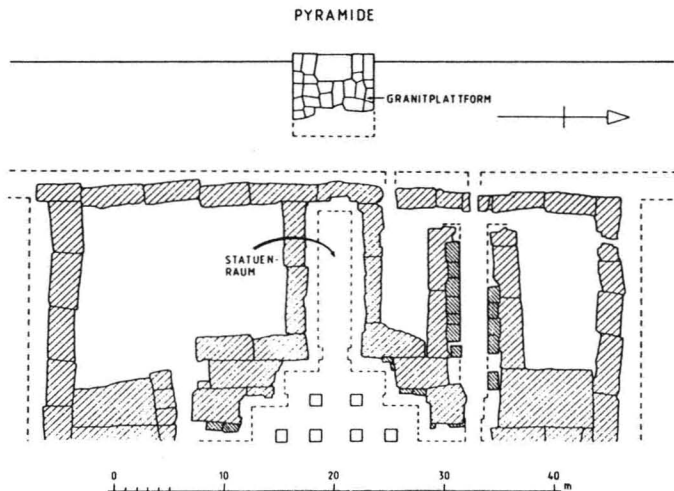
Abb.4 Der westliche Teil des Mykerinostempels (nach MARAGIOGLIO/RINALDI, L'architettura VI, Tf.8 Fig.1)
