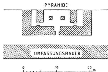
Abb.6 Die Kultkapelle an der Ostseite der Userkafpyramide (nach MARAGIOGLIO/RINALDI, L'architettura VII, Tf.1 Fig.1)
